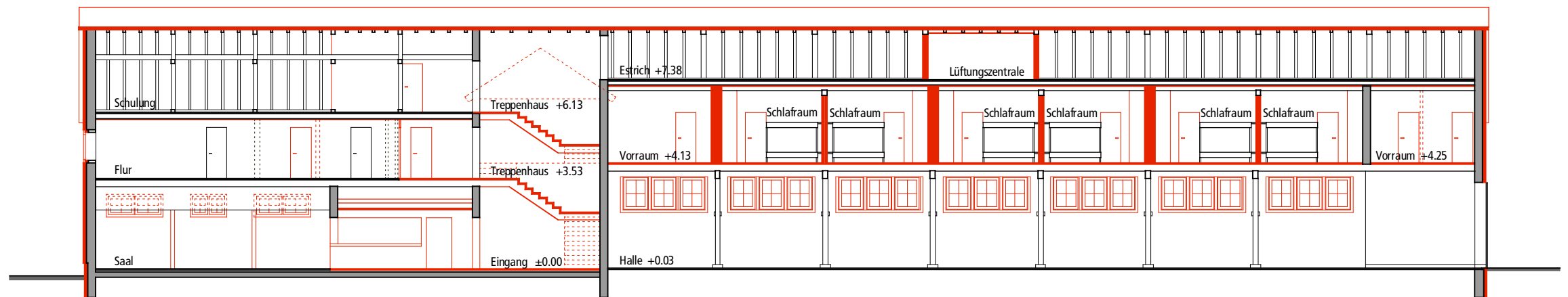
Schnitt C
