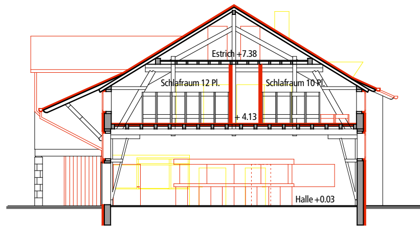
Schnitt A
