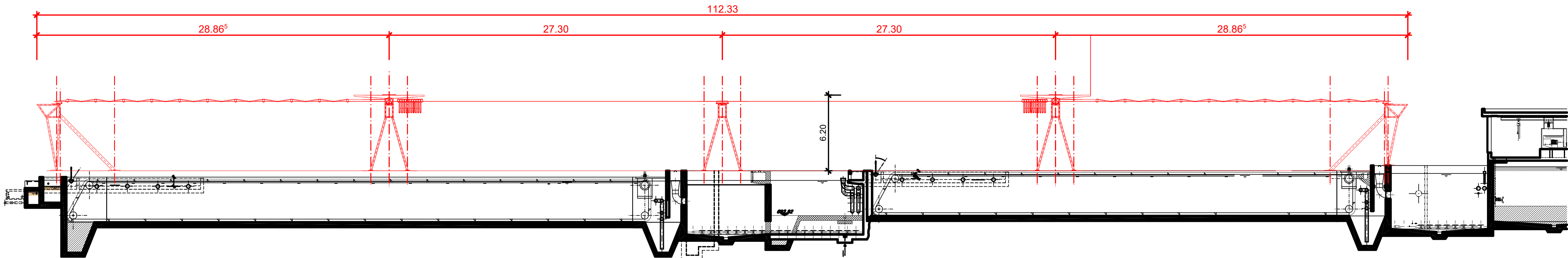
Längsschnitt 1-1 1:200
