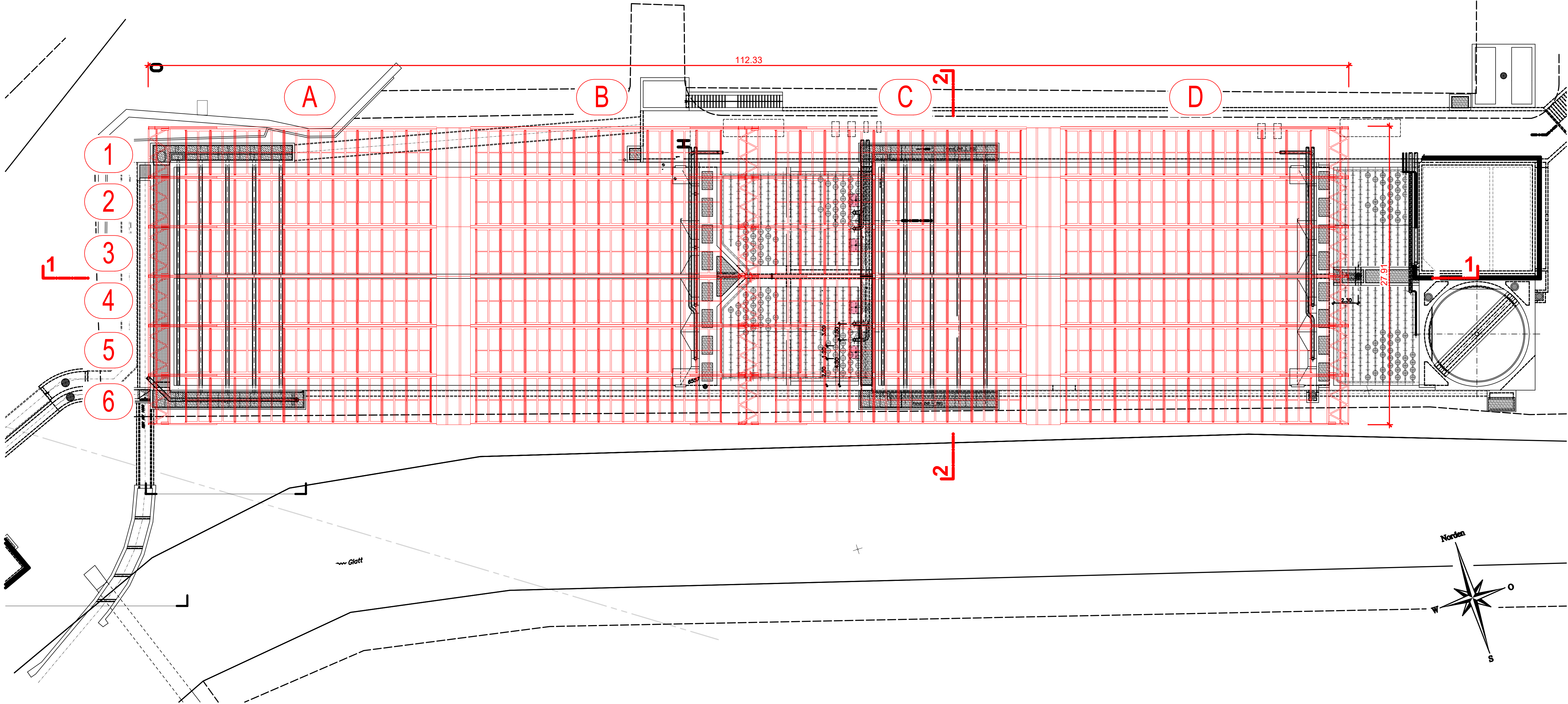
Grundriss 1:200
